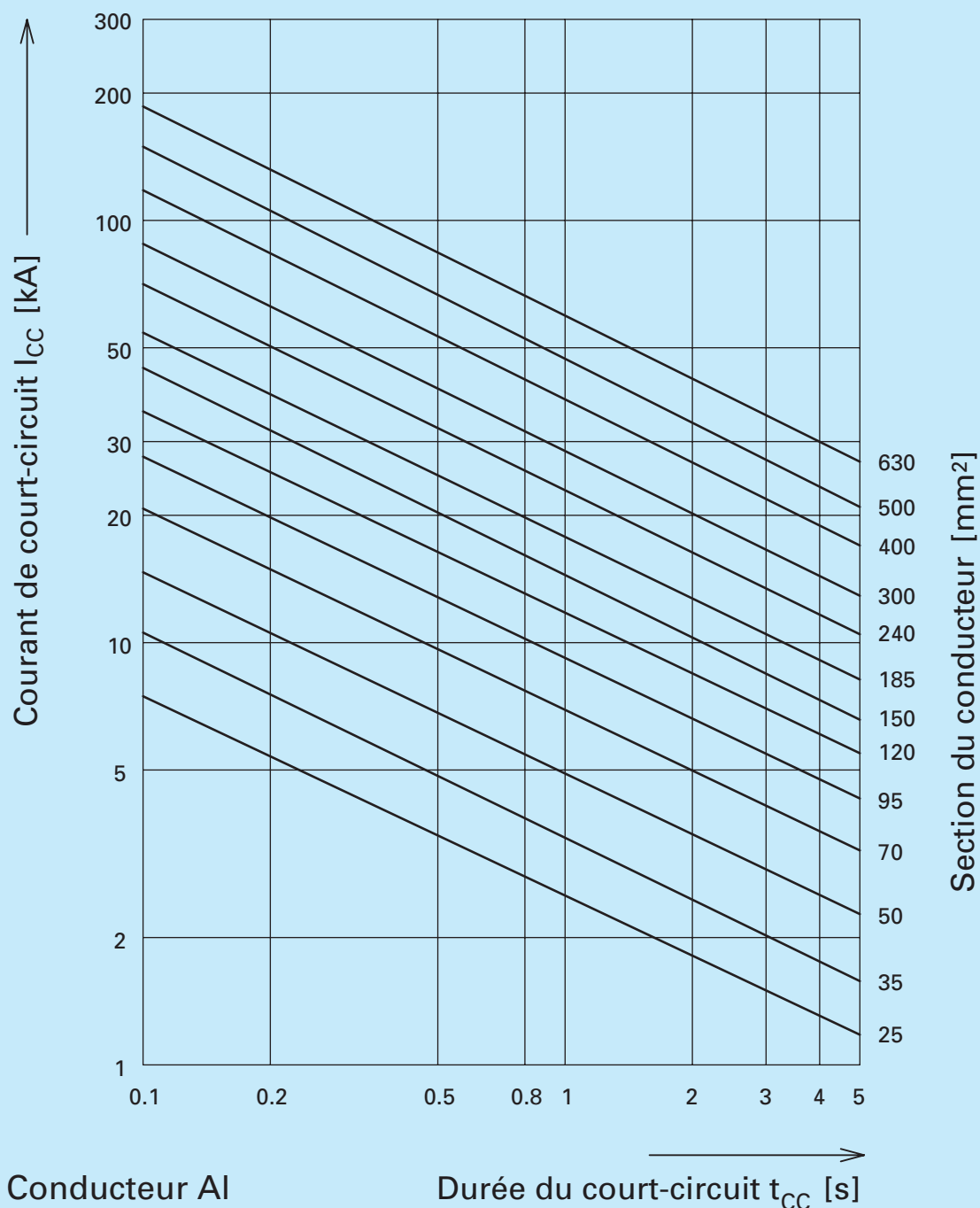
Figure 4: Détermination des courants de courts-circuits autorisés pour les conducteurs en aluminium.
